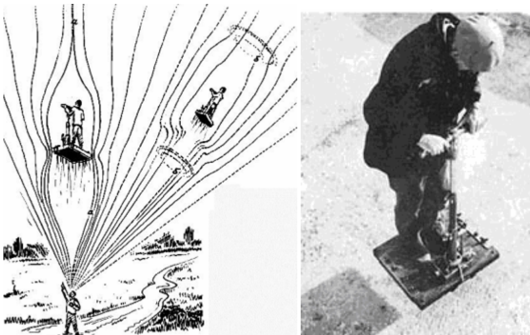
Рис. 4-6-1. Причины эффекта невидимости гравитоплана.
